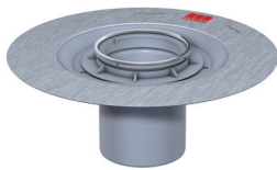
Corp superior rotund cu flanșă de impregnare
