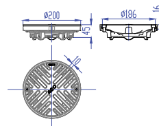
Art.no. 7000.08.02 Ramă cu grătar Diametru: 200 mm Clasă de sarcini: M125
