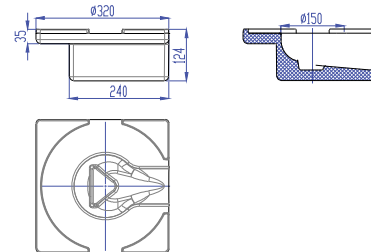
Art.no. 7040.34.02 Corp izolator Material: Poliuretan
