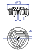
Art.no. 7000.10.02 Parfrunzar Diametru: 215 mm
