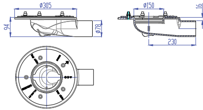
Art. no. 7047.10.22 Extensie din fontă
