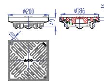
Art.no. 7000.44.02 Ramă cu grătar Dimensiuni: 200 x 200 mm Clasă de sarcini: M125
