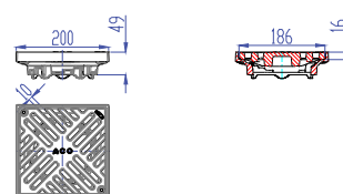
Art.no. 7000.44.02 Ramă cu grătar Dimensiuni: 200 x 200 mm Clasă de sarcini: M125
