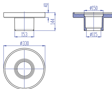
Art.no. 7040.21.02 Corp izolator Material: Poliuretan
