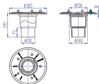
Art. no. 7034.10.12 Corp inferior din fontă
