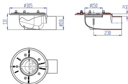
Art. no. 7054.11.12 Corp inferior din fontă
