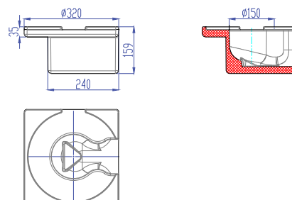
Art.no. 7040.31.02 Corp izolator Material: Poliuretan
