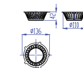
Art.no. 7000.03.02 Coș de aluviuni
