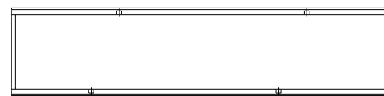
Element de rigolă cu înălțime redusă, fără pantă prefabricată, cu garnitură de etanșare DN100 pentru descărcare verticală, L=1m
