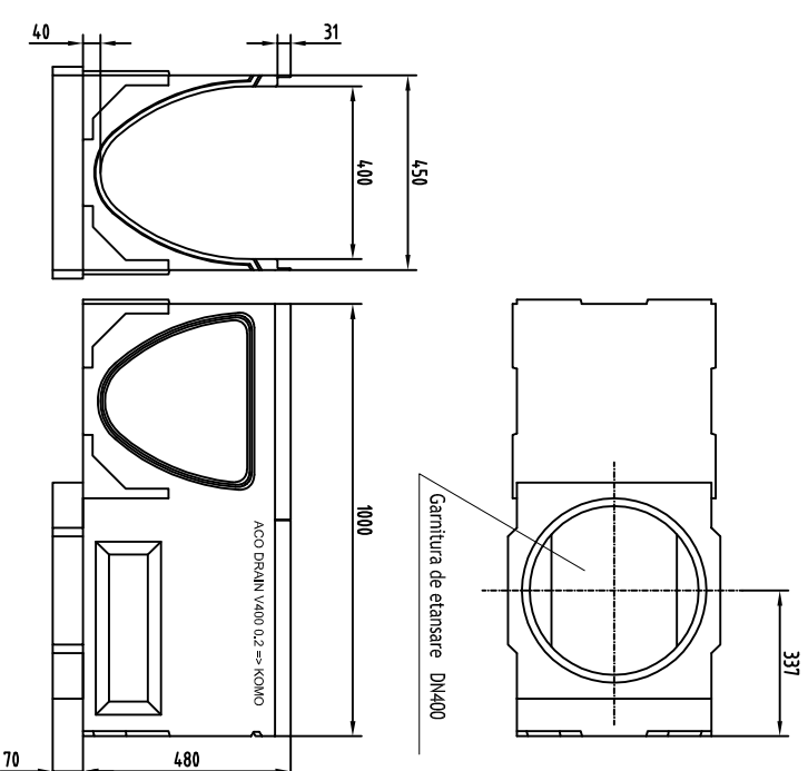
Element de rigola fara panta prefabricata, cu garnitura verticala de etansare DN400, L=1m
