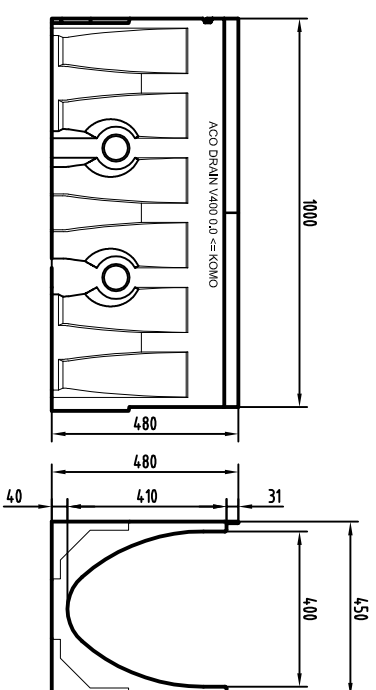
Element de rigola fara panta prefabricata, L=1m
