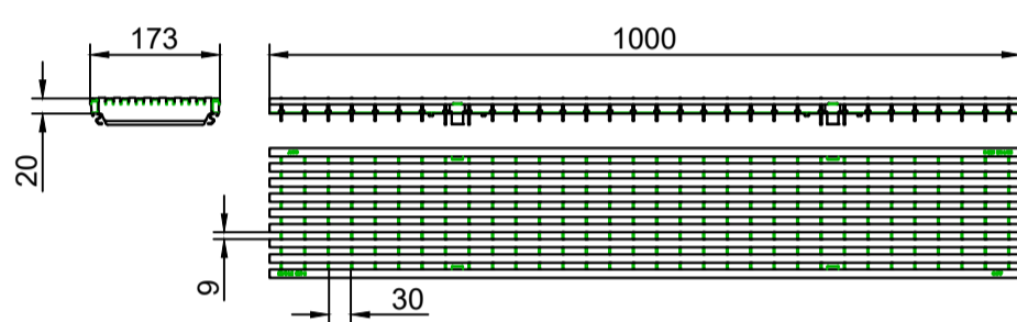
Gratar nervurat longitudinal, clasa de sarcini B125
