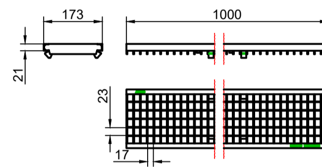
Gratar retea Q*, clasa de sarcini C250
