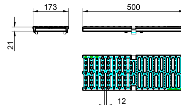
Gratar nervurat transversal din fonta, clasa de sarcini C250
