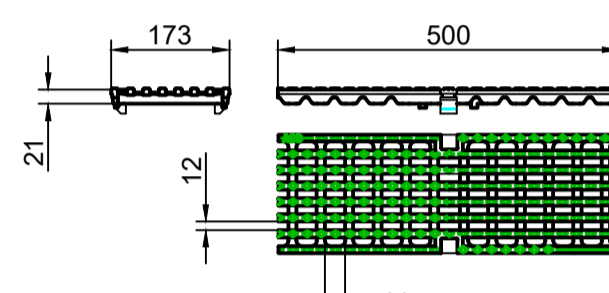
Gratar nervurat longitudinal, clasa de sarcini C250
