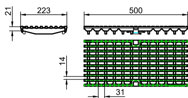
Gratar nervurat longitudinal, clasa de sarcini C250
