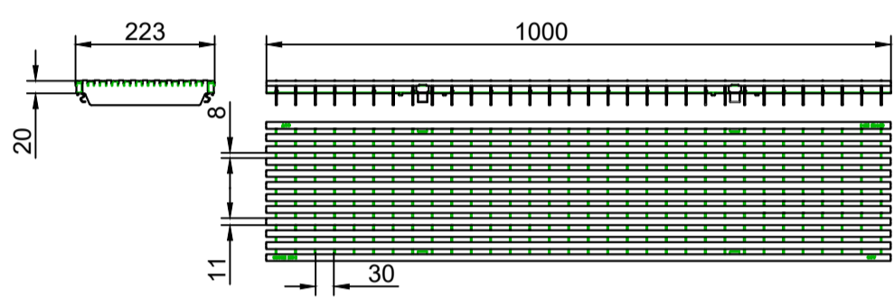
Gratar nervurat longitudinal, clasa de sarcini B125
