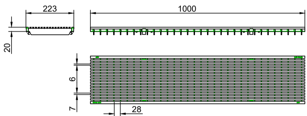
Gratar nervurat longitudinal pentru protectia tocurilor, clasa de sarcini B125
