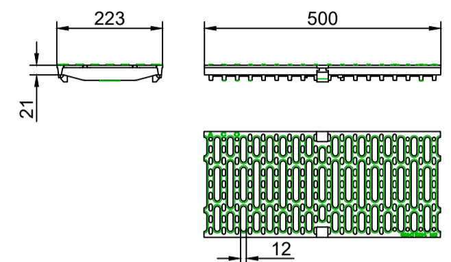
Gratar nervurat transversal, clasa de sarcini D400
