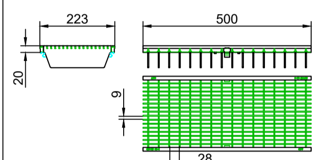
Gratar retea Q*, clasa de sarcini D400
