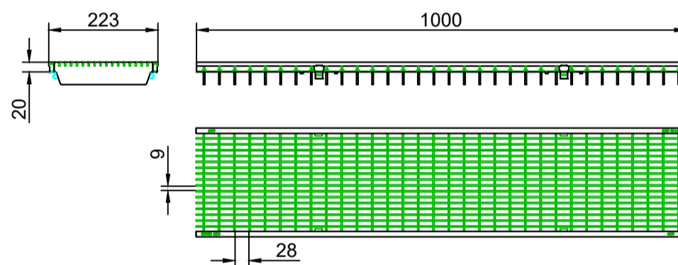
Gratar retea Q*, clasa de sarcini C250
