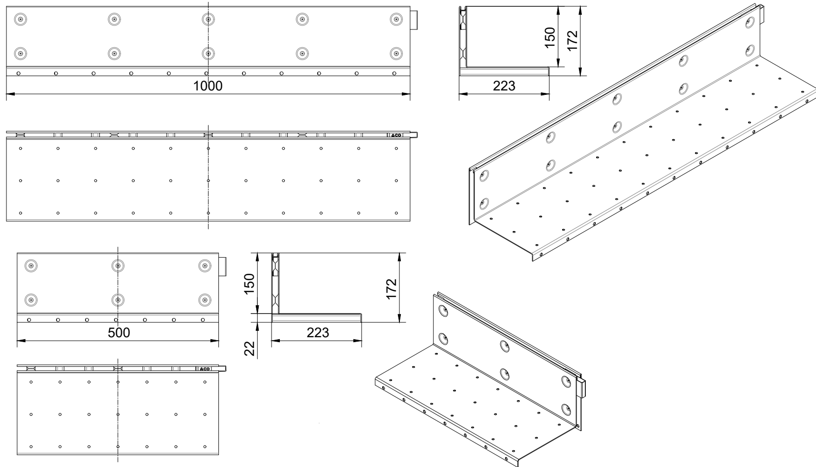
Gătare SlotTop L= 1000 mm/500 mm
