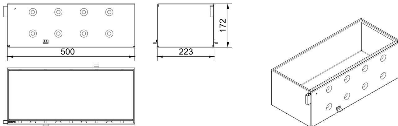
Element de revizie L= 500 mm
