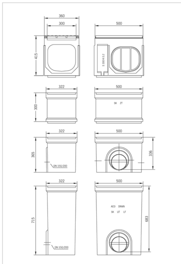
Cămin colector S 300 K
