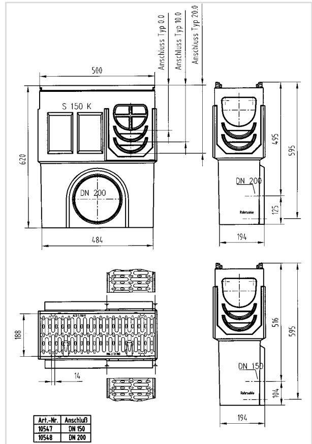
Cămin colector S 150 K
