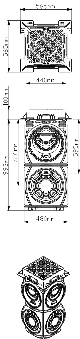
Cămin de descărcare cu ramă și grătar D400, art. 32972 Detaliu montaj - planșa 21983
