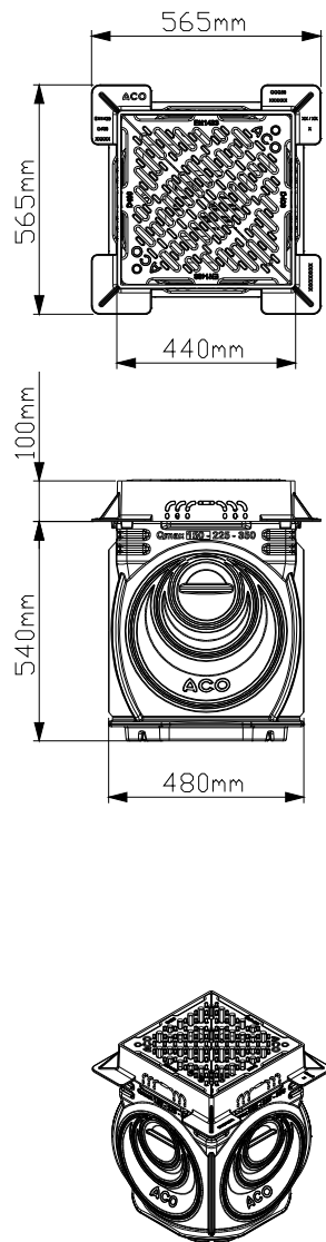
Cămin de acces cu ramă și grătar D400, art. 32970 Detaliu montaj - planșa 21981
