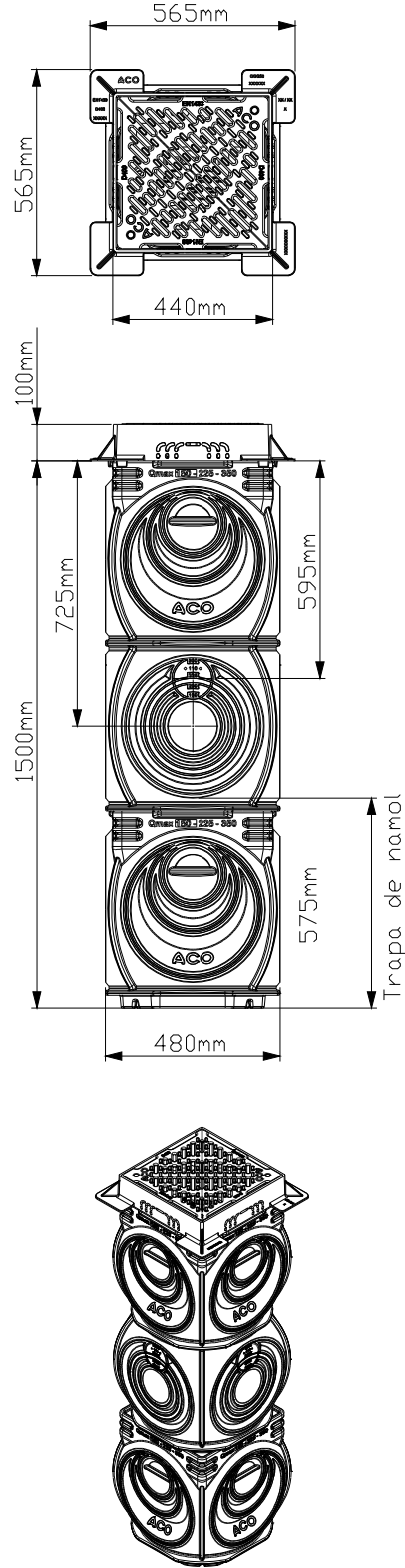
Cămin de descărcare cu ramă și grătar D400 și trapă de nămol, art. 32974 Detaliu montaj - planșa 21985
