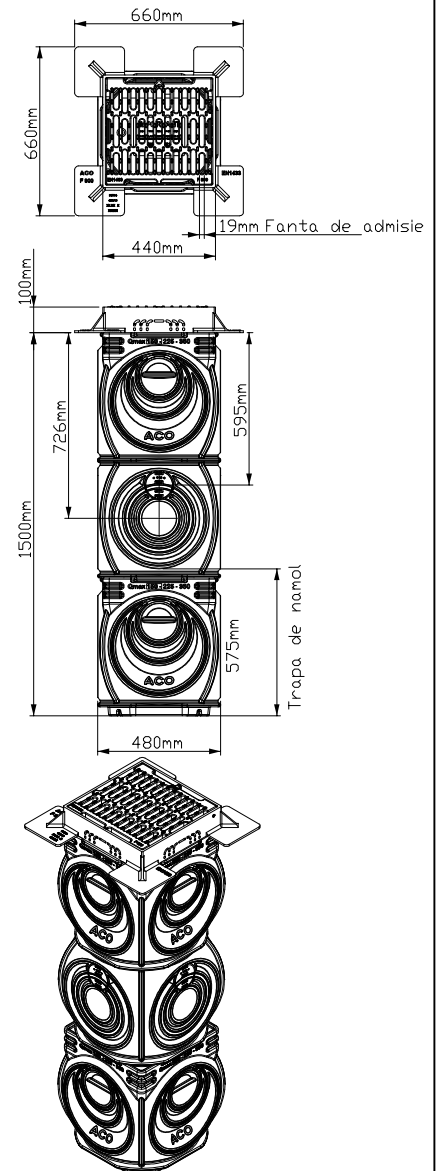
Camin de descarcare rama si gratar D400/F900
