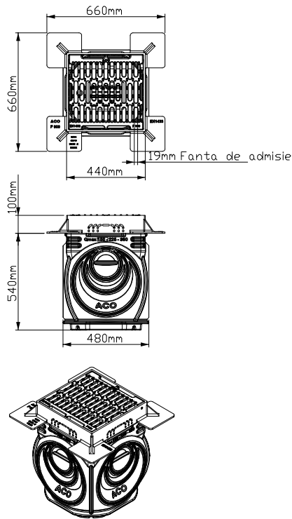
Camin de acces cu rama si gratar D400/F900
