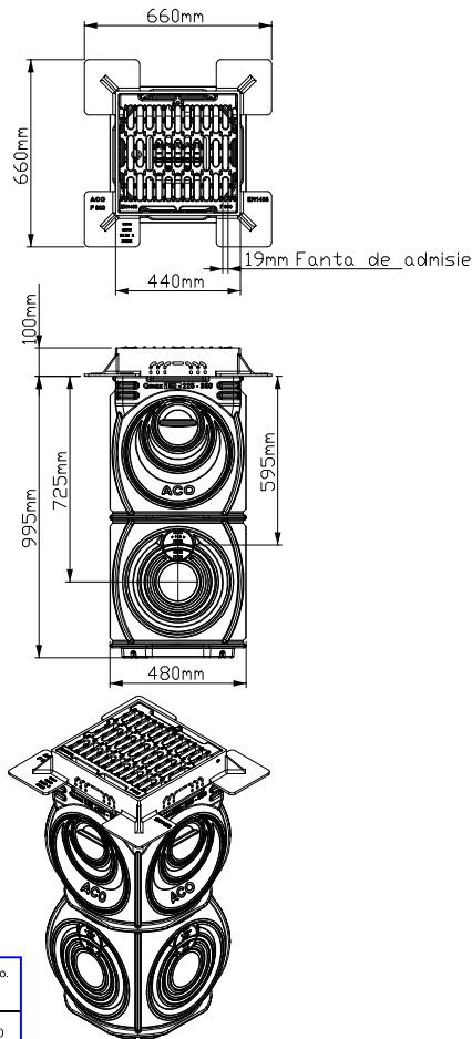
Camin de descarcare cu rama si gratar D400/F900
