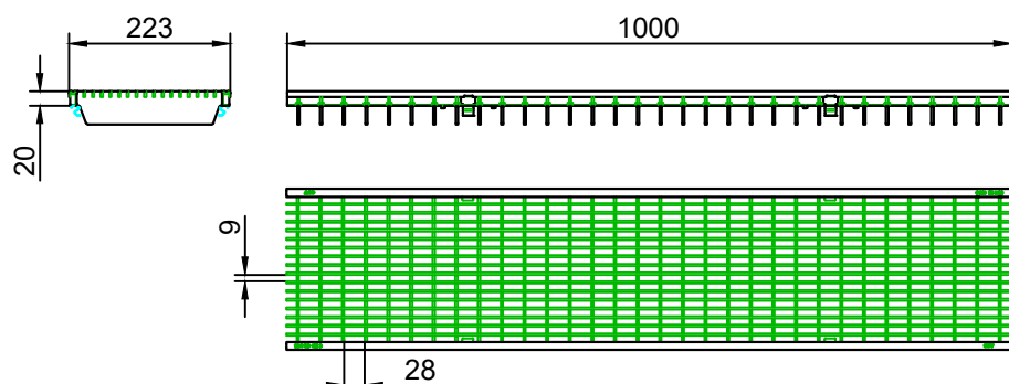
Gratar retea Q*, clasa de sarcini C250
