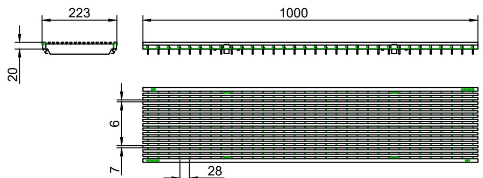
Gratar nervurat longitudinal pentru protectia tocurilor, clasa de sarcini B125
