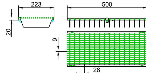
Gratar retea Q*, clasa de sarcini D400
