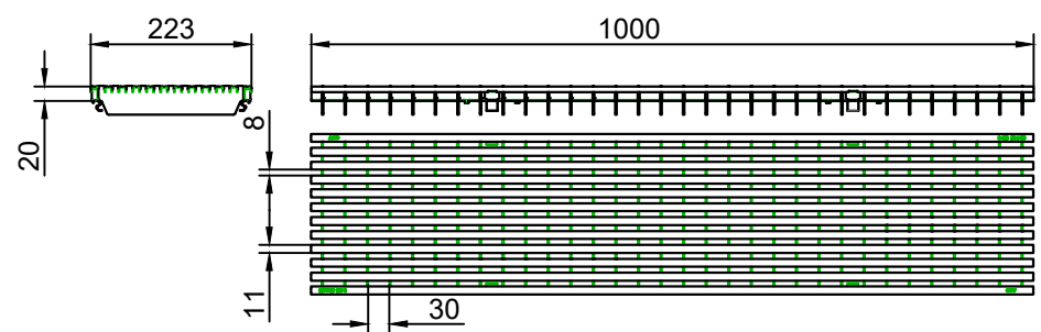
Gratar nervurat longitudinal, clasa de sarcini B125
