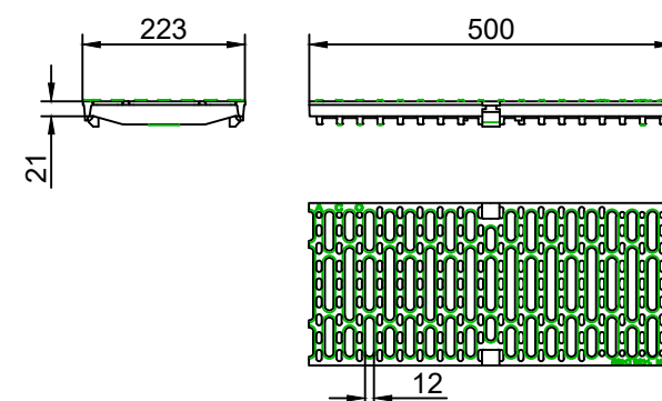
Gratar nervurat transversal, clasa de sarcini D400/E600
