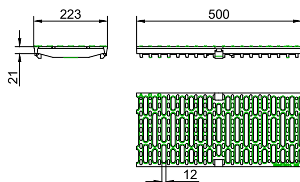
Gratar nervurat transversal, clasa de sarcini D400
