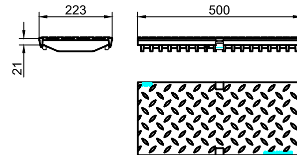
Placa de acoperire, clasa de sarcini E600
