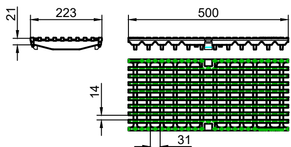
Gratar nervurat longitudinal, clasa de sarcini C250
