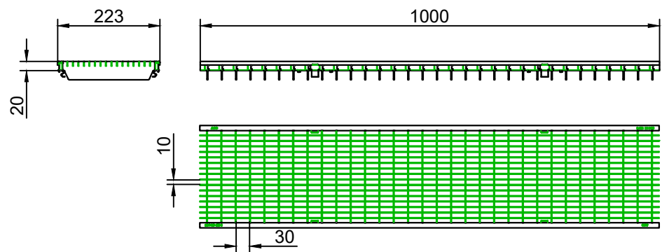
Gratar retea Q*, clasa de sarcini B125
