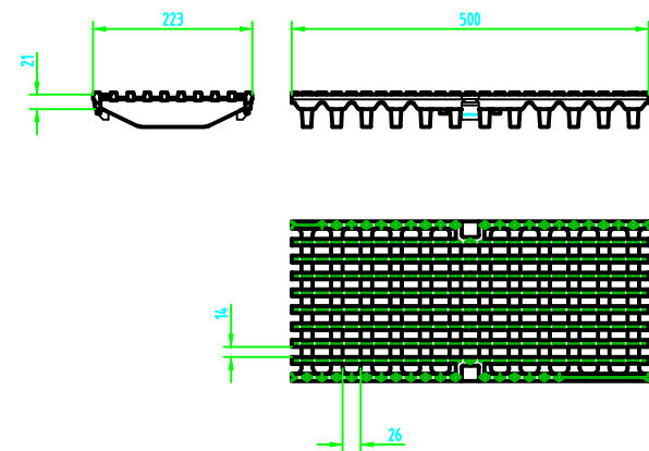
Gratar nervurat longitudinal, clasa de sarcini D400/E600
