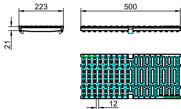
Gratar nervurat transversal din fonta, clasa de sarcini C250
