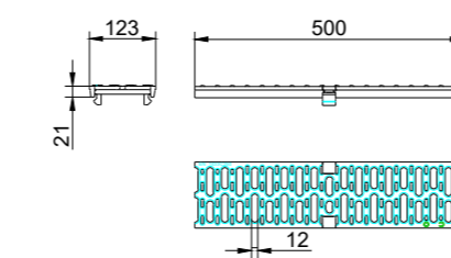
Grătar nervurat transversal, clasă de sarcini C250
