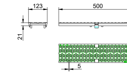
Grătar nervurat transversal pt protecția tocurilor, clasă de sarcini C250
