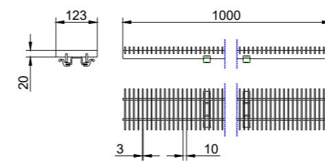
Grătar cu bare transversale, clasă de sarcini B125
