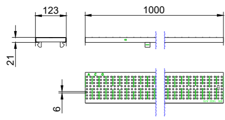
Grătar cu bare perforate, clasă de sarcini A15
