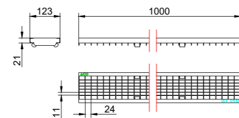
Grătar rețea Q*, clasă de sarcini B125
