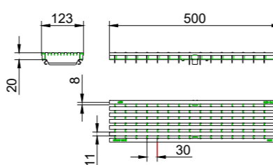
Grătar nervurat longitudinal, clasă de sarcini B125
