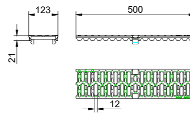
Grătar nervurat transversal, clasă de sarcini B125
