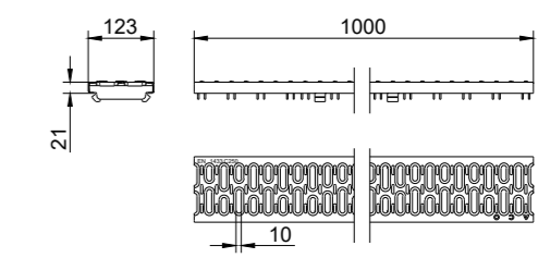
Grătar nervurat transversal, clasă de sarcini D400
