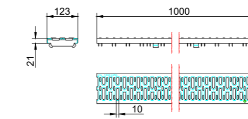
Grătar nervurat transversal, clasă de sarcini C250
