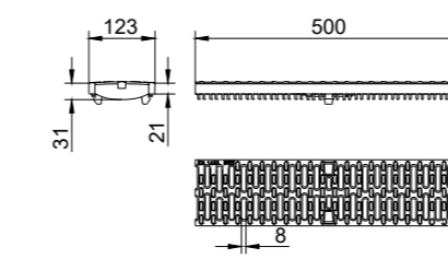
Grătar din polipropilenă cu Microgrip, clasă de sarcini B125
