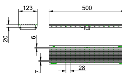
Grătar nervurat longitudinal pentru protecția tocurilor, clasă de sarcini B125
