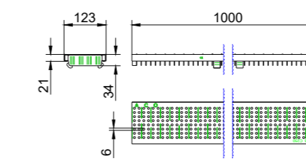
Grătar perforat, clasă de sarcini C250
