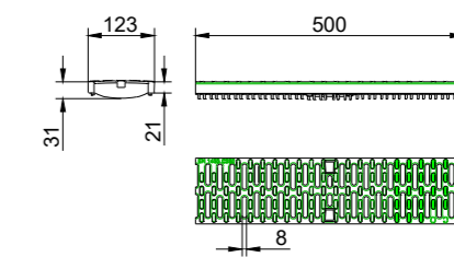
Grătar din polipropilenă cu Microgrip, clasă de sarcini C250
