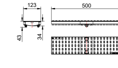
Placă de acoperire, clasă de sarcini B125
