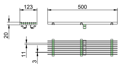
Grătar cu bare longitudinale, clasă de sarcini A15
