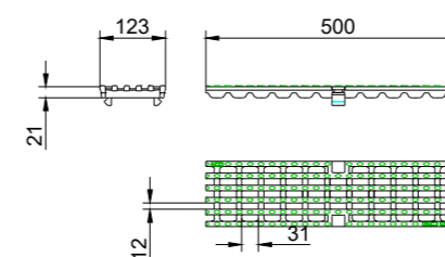
Grătar nervurat longitudinal, clasă de sarcini C250
