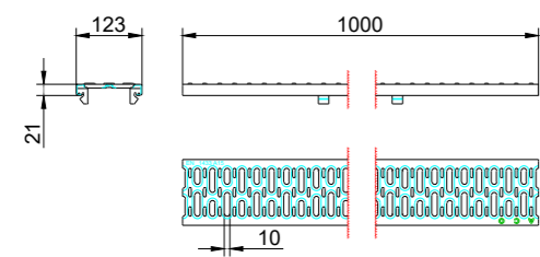
Grătar nervurat transversal, clasă de sarcini A15
