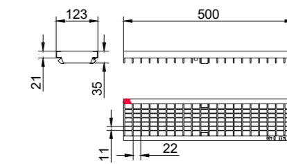
Grătar rețea Q*, clasă de sarcini D400
